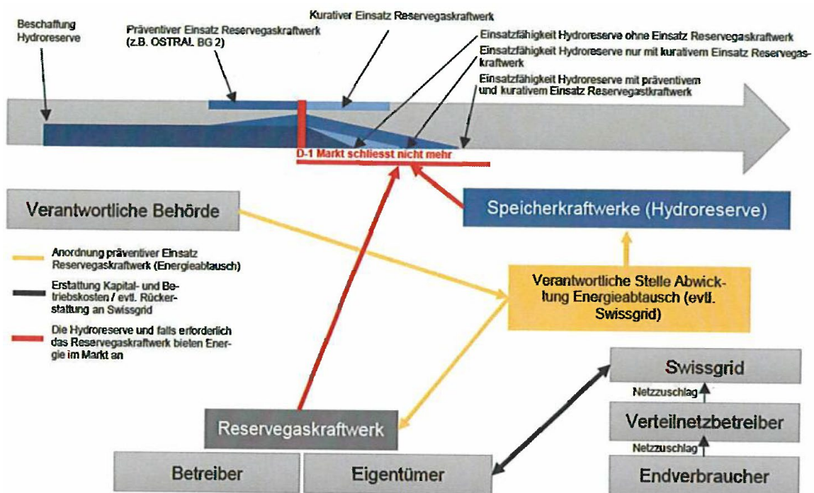
Abbildung 5: Akteure und Rollen bei der Kombination von Hydroreserve und Reservegaskraftwerken (ECom, 2021b). Die ECom empfiehlt den präventiven Einsatz der Reservegaskraftwerke zur Schonung der Hydroreserve, damit die Reservegaskraftwerke kleiner dimensioniert werden können.
